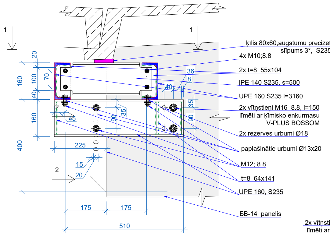
Mezglis D M 1:10
