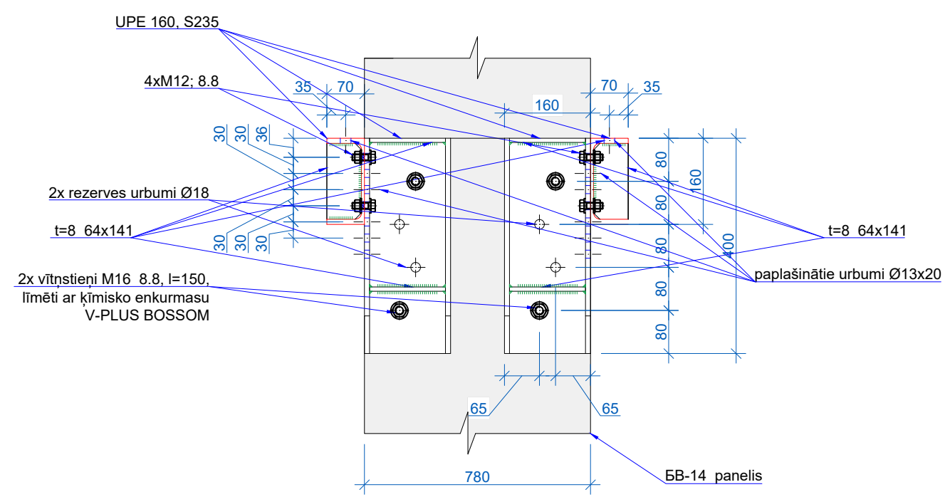
2 - 2 M 1:10
