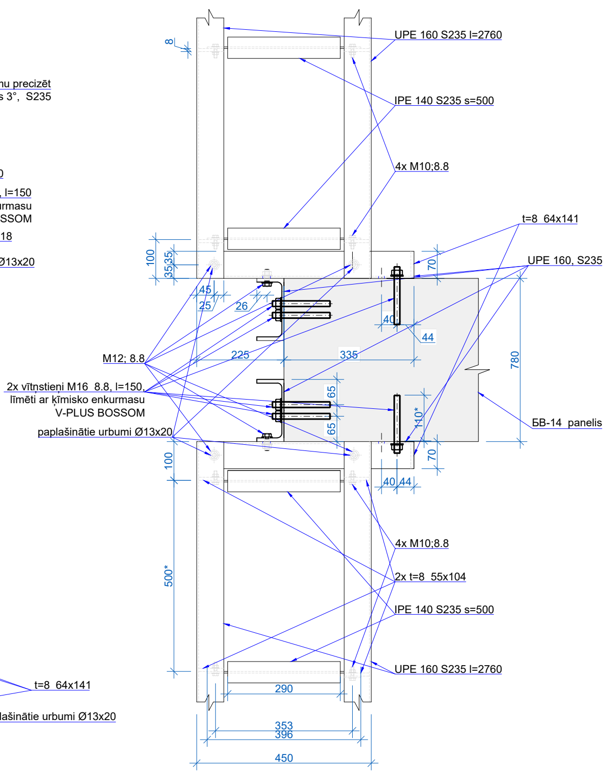
1 - 1 M 1:10
